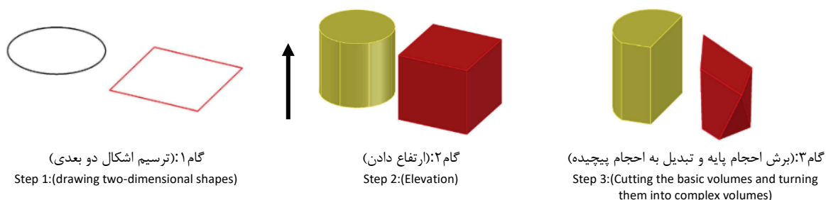
شکل ۳: گام‌های مدل‌سازی اجسام پیچیده از نگاه دانش‌آموزان Fig. 3: The steps of modeling complex volumes from the perspective of students
