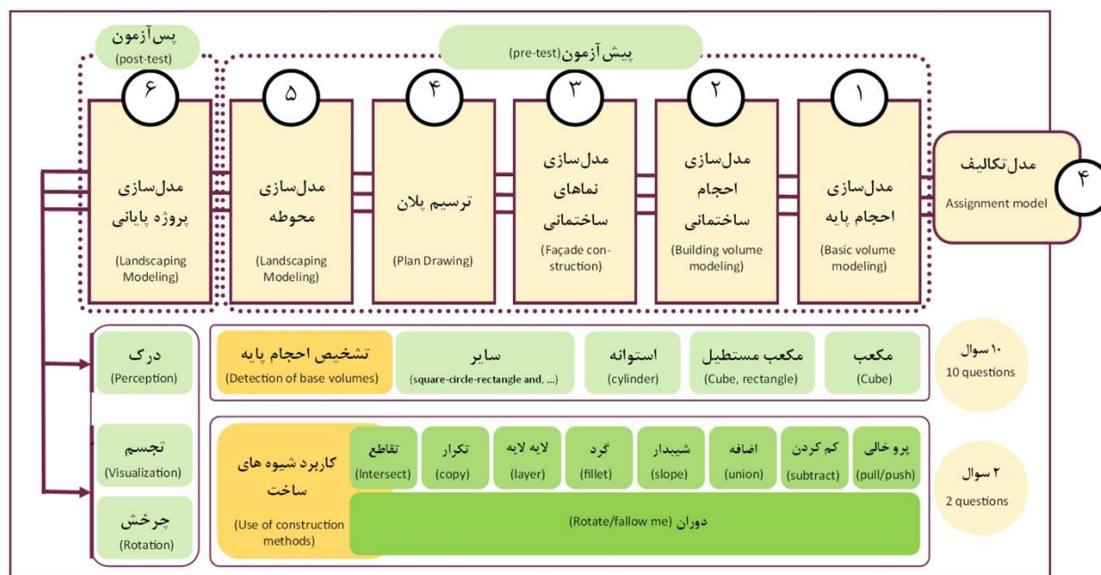
شکل ۲: روابط بین پیش آزمون و پس آزمون ها با تکالیف درسی Fig. 2: Relationships between pre-test and post-tests with homework
