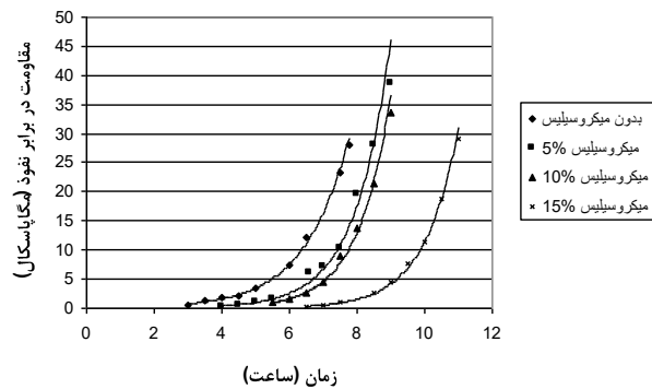
شکل ۱ مقاومت در برابر نفوذ بتن
