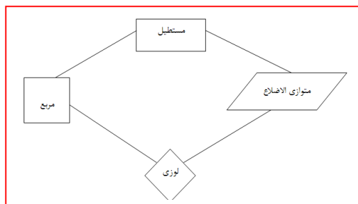
شکل 4 مثالی از مرتب سازی متوازی‌الاضلاع‌ها (هالت، 2008)
