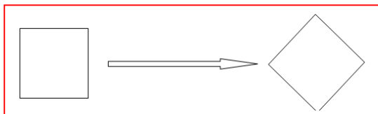
شکل 2 دوران مربع به اندازه 45 درجه
