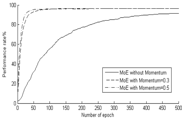
شکل ۷ نمودار نرخ بازشناسی چهره بر حسب تعداد تکرارهای آموزش ساختار بر روی بانک چهره ORL
