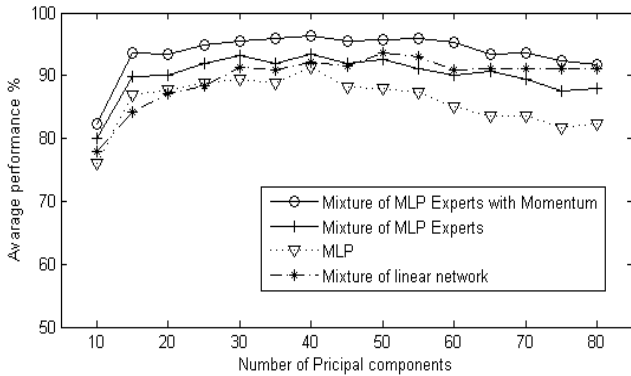
شکل ۴ کارایی سیستم نسبت به تعداد مؤلفه های اساسی
