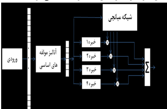
شکل ۵ ساختار ارایه شده مبتنی بر اختلاط خبره ها و نحوه بازنمایی تصاویر چهره به خبره ها و شبکه میانجی
