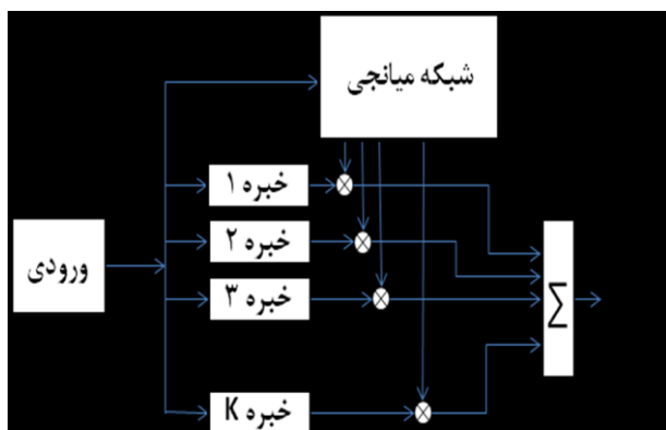
شکل ۱ ساختار مدل اختلاط خبره ها
