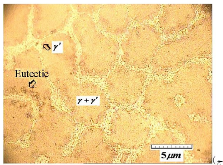
شکل ۲ تصویر میکروسکوپ نوری (الف) نمونه ریختگی (ب) نمونه کار گرم شده HP 4 (ب) و (ج) نمونه پرس گرم دو مرحله‌ای HP 6
