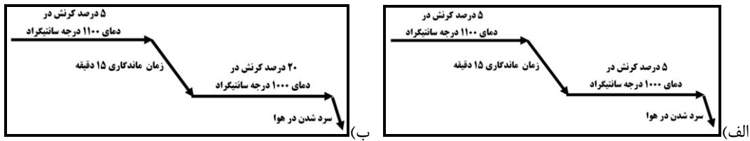
شکل ۱ شرایط اعمال فرآیند پرس گرم دو مرحله‌ای HP5 (الف) و HP6 (ب) با نرخ کرنش 1/s
