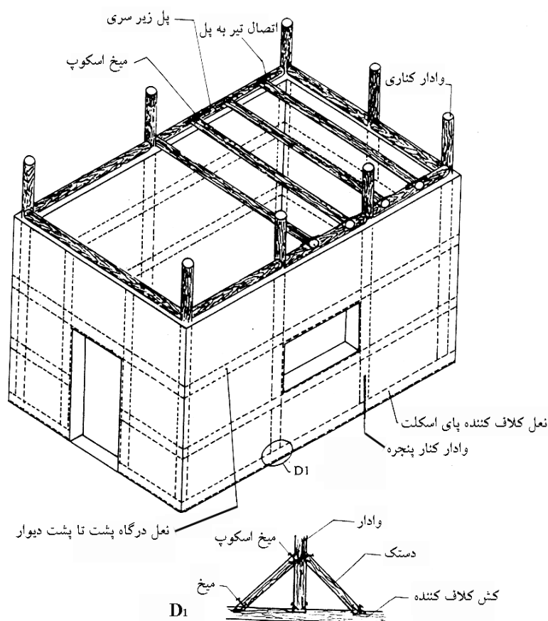
شکل ۵ کلافبندی افقی و عمودی در نبش در، دربند و ... جهت ضد زلزله
