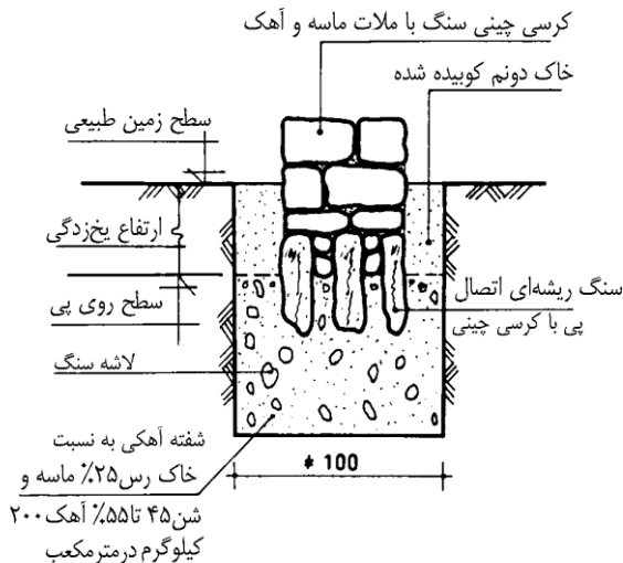
شکل ۲ جزئیات پی سازی سنتی (شفته‌ای)
